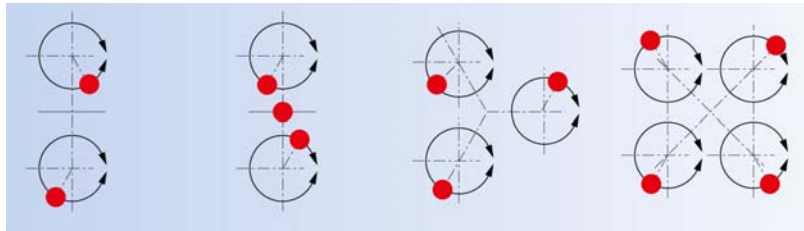
Abb. 3: Bohrbilder bei verstellbaren Köpfen mit 2, 3 oder 4 Spindeln
