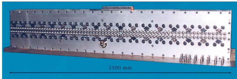
Fig. 4: Cabezal múltiple POLYdrill con 144 husillos a distancias fijas entre ejes
