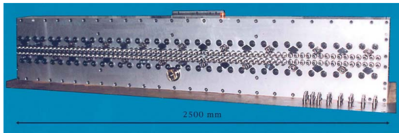
vue 4 : tête POLYdrill à entraxes fixes avec 144 broches
