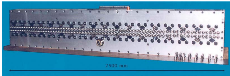
Fig. 4: Testa multipla POLYdrill a interasse fisso, fino a 144 alberi
